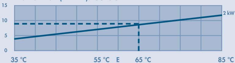
Aufheizzeit (in min): CUN 5
