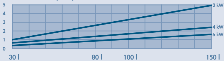
Aufheizzeit (in h) bis 65 °C: CWD
